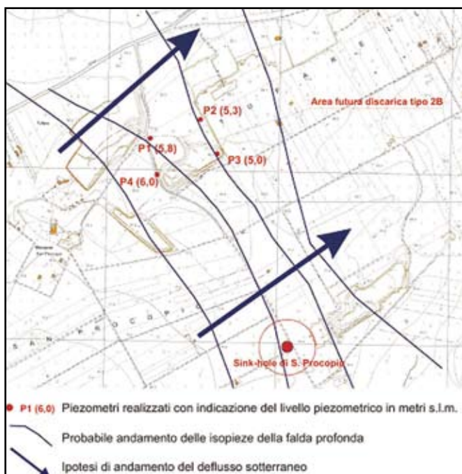
Fig. 2 - Caratteri idrogeologici dell'area di studio. Fig. 2 - Hydrogeological features of the study area.
