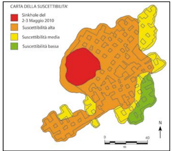
Fig. 9 - Zonazione preliminare della suscettibilità. Fig. 9 - Preliminary susceptibility zonation.
